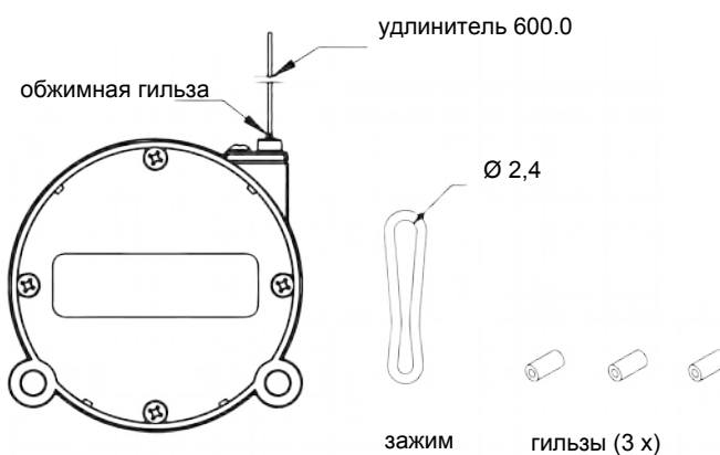
удлинитель троса с гильзами
